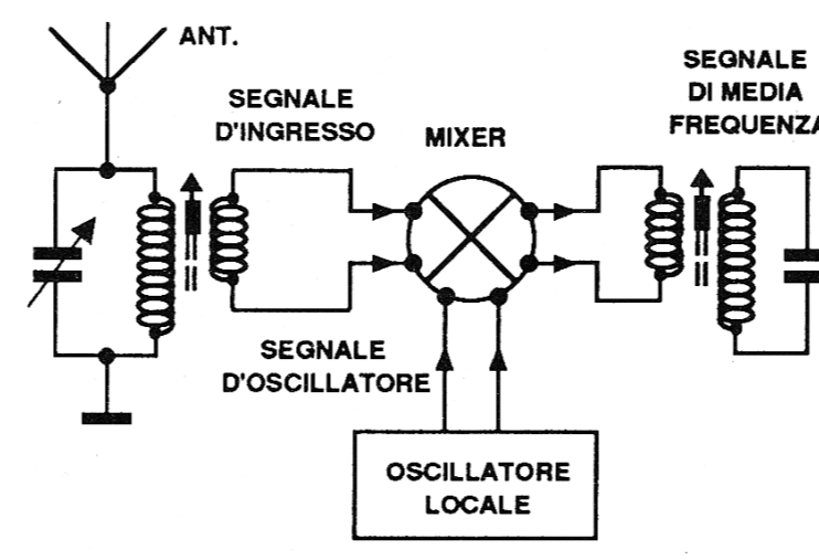
Schema a blocchi di un convertitore RF.
